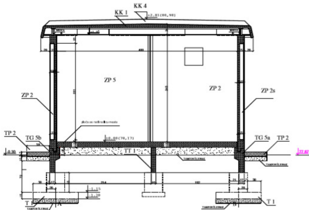
Presek A - A , TP 45A
