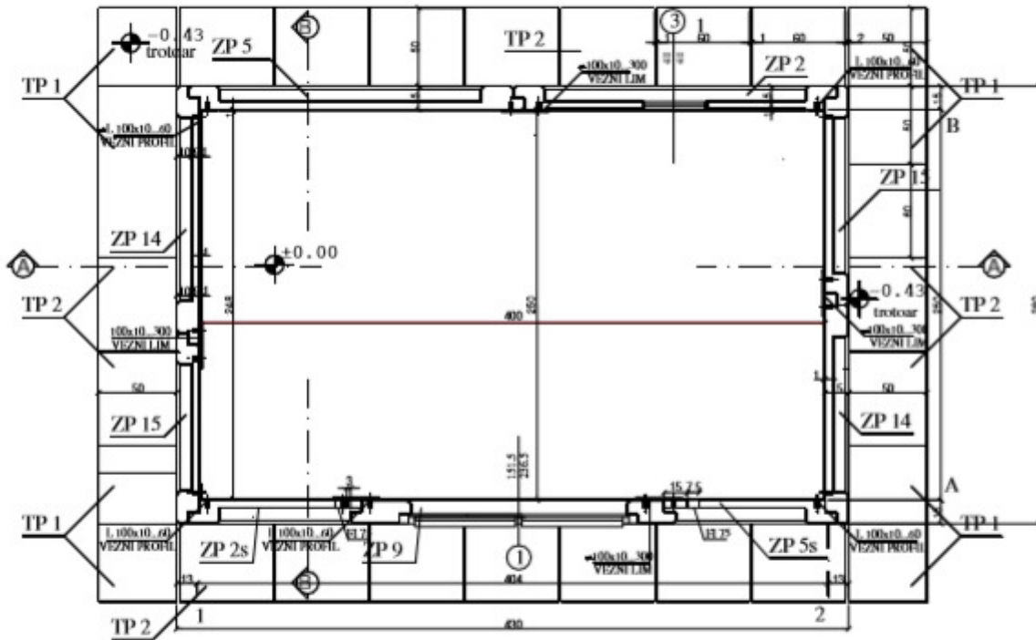
osnova prizemlja TP BP 19
