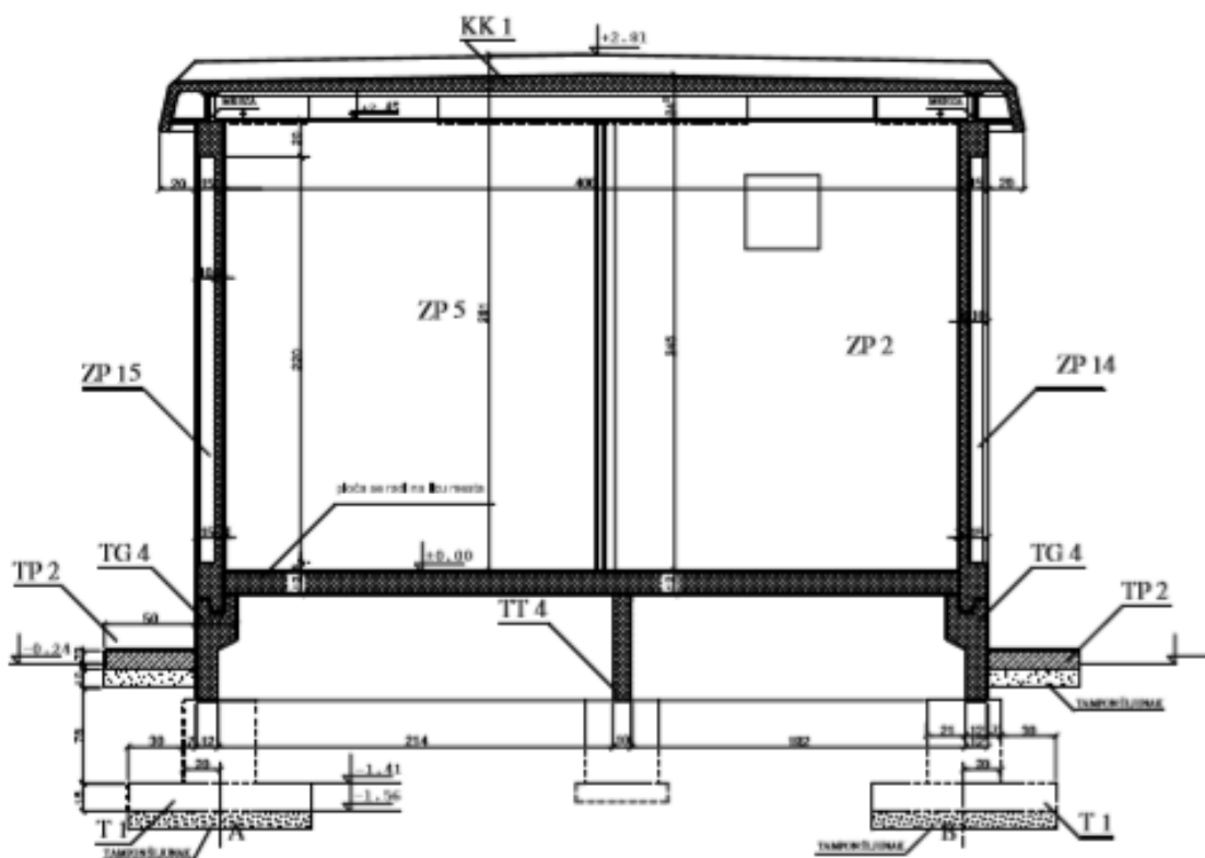
presek A - A, TP BP 19
